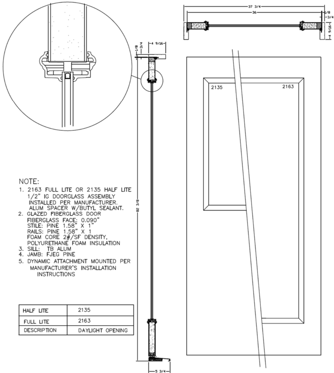
3068 DASD REFERENCE FIBERGLASS DOOR
