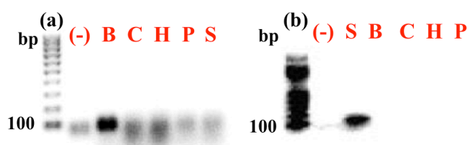
Figure 1. (a) B. bruxellensis -specific PCR (b) S. cerevisiae -specific PCR (-): negative control, B: B. bruxellensis , C: Candida apicola , H: H. osmophilla , P: P. membranifaciens , S: S. cerevisiae
