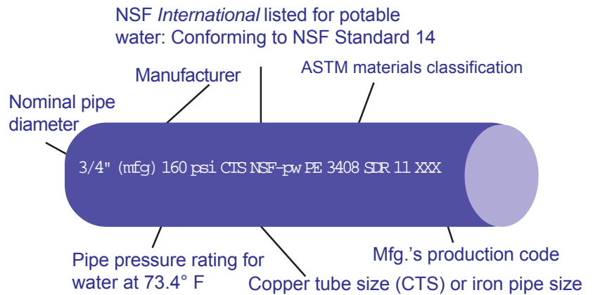
Figure 1: PE pipe markings
